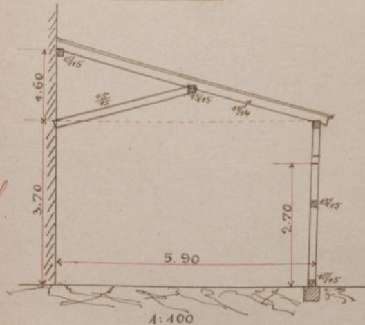
Metszet.
